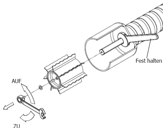
Abb. 3 Walzen wechseln
